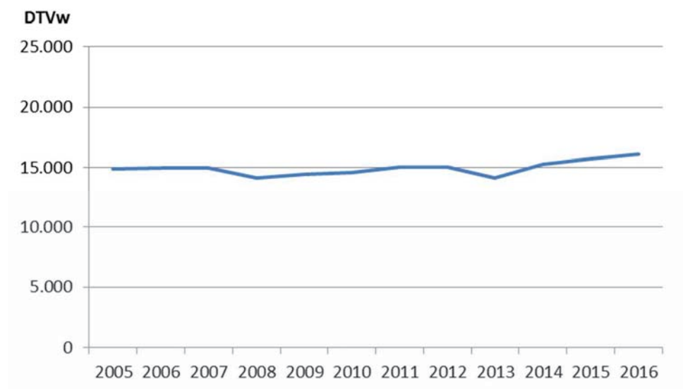
Abb. 4 Werk tägliche Verkehrsstärken ( DTV_{w5} ) am Querschnitt Hofweg südlich der Körnerstraße in den Jahren 2005 bis 2016
